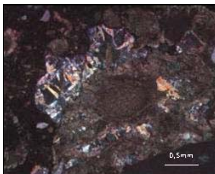
fig 7. Desarrollo de sales de yeso y anhídrita en el frente de sales. Microscopia óptica. NC.
