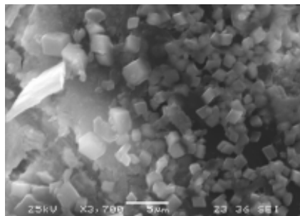
fig 8. Desarrollo de halita con hábito cúbico sobre la capa ocre. SEM-se.
