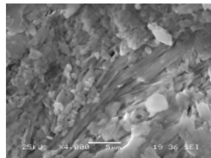
fig 9. Desarrollo de cristales de halita de hábito fibroso en el frente de sales. SEM-se.
