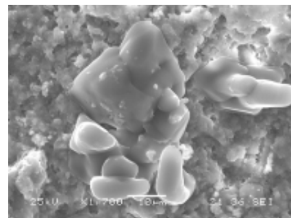
fig 10. Sales de Natrón, SEM - se.
